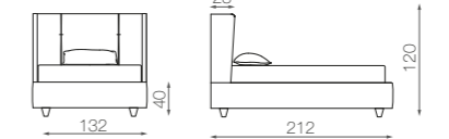
RITZ 120 - mat. 120 x 195
