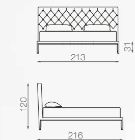
RETE 200X200 MAT. 200X200 LETTO 200 / BED 200
