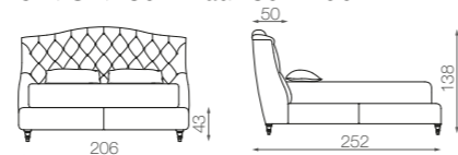
SAVON 180 - mat. 180 x 200
