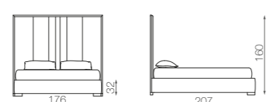
SEINE 160 - mat. 160 x 195
