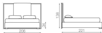
DIAMOND 180 - mat. 180 x 200
