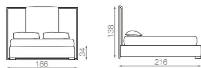
DIAMOND 160 - mat. 180 x 195
