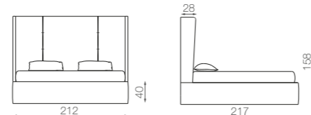
MAISON 200 - mat. 200 x 200
