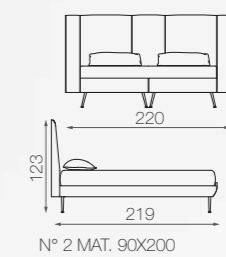
LETTO TWIN / TWIN BED
