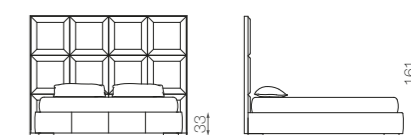
QUINN 180 - mat. 180 x 200
