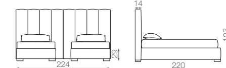
MILANO TWIN - mat. n°2 90 x 200
