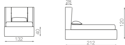
MAISON 120 - mat. 120 x 195
