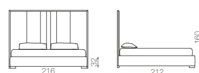
SEINE 200 - mat. 200 x 200
