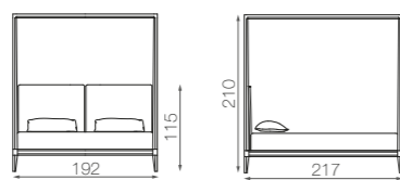
ASPEN CANOPY 180 - mat. 180 x 200
