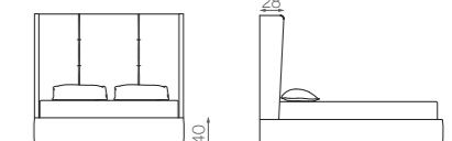
RITZ 160 - mat. 160 x 195
