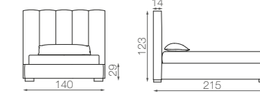
MILANO 120 - mat. 120 x 195
