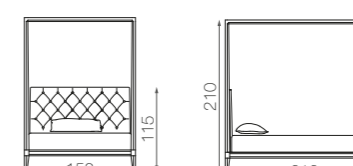
CORTINA CANOPY 140 - mat. 140 x 195
