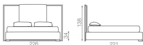
DIAMOND 200 - mat. 200 x 200
