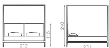
ASPEN CANOPY 200 - mat. 200 x 200
