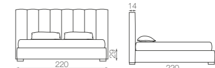
MILANO 200 - mat. 200 x 200
