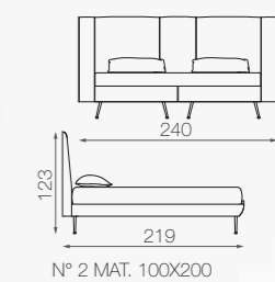
LETTO TWIN / TWIN BED
