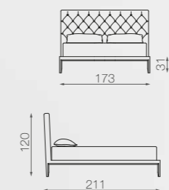
RETE 160X195 MAT. 160X195 LETTO 160 / BED 160
