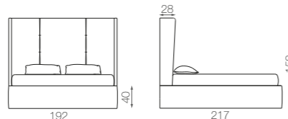
MAISON 180 - mat. 180 x 200
