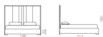
SEINE 180 - mat. 180 x 200
