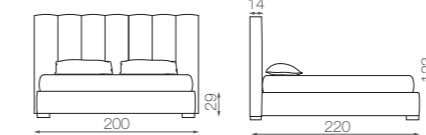
MILANO 180 - mat. 180 x 200
