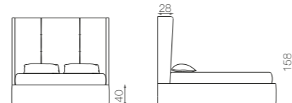
MAISON 160 - mat. 160 x 195
