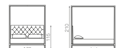
CORTINA CANOPY 160 - mat. 180 x 195
